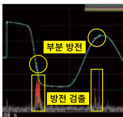
방전검출기능 ST9000
