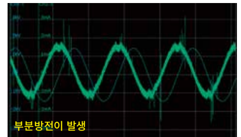
유사 불량품의 AC1.0kV 인가 시의 전류·전압파형
