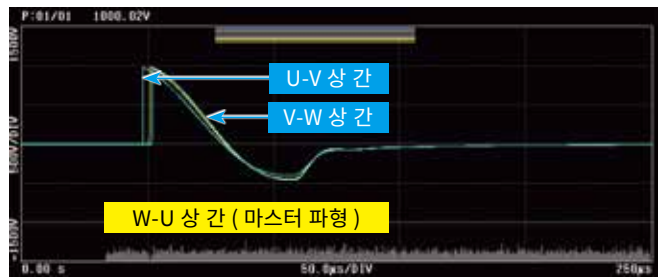
양품의 응답파형
